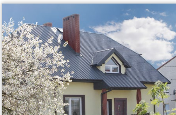
Profil T20 – blacha trapezowa. Zastosowanie: pokrycie dachowe. Wysokość całkowita [mm]: 17. Szerokość efektywna [mm]: 1095. Szerokość całkowita [mm]: 1129. Min. dł. [mm]: 600. Maks. dł. [mm]: 12 000. Wykończenie powierzchni: powłoka Pural mat, Poliester, Poliester mat, Purex. Kolory: czarny, grafitowy, ciemny brąz, czekoladowy brąz, ceglasty, wiśniowy, zielony, biały, srebrny. Gwarancja: 50 lat techniczna i 20 lat estetyczna.
